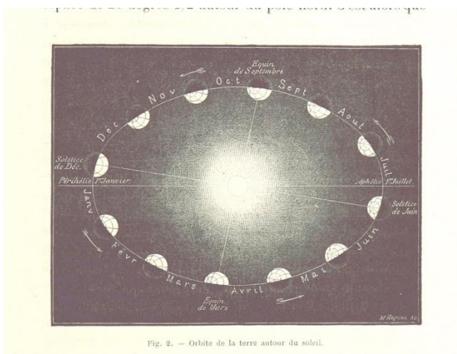
Fig. 2. — Orbite de la terre autour du soleil.
